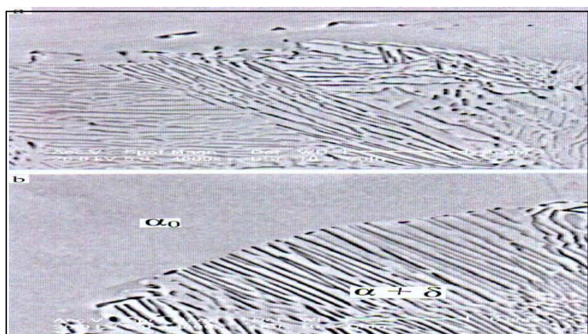
Figure 2. Deux types de cellules: (a) cellules caractérisées par une distance interlamellaire irrégulière (b) colonie idéale de précipité discontinu lors du vieillissement isotherme de l'alliage Cu-7,5 at. % In a 400°C pendant 12 heures.
