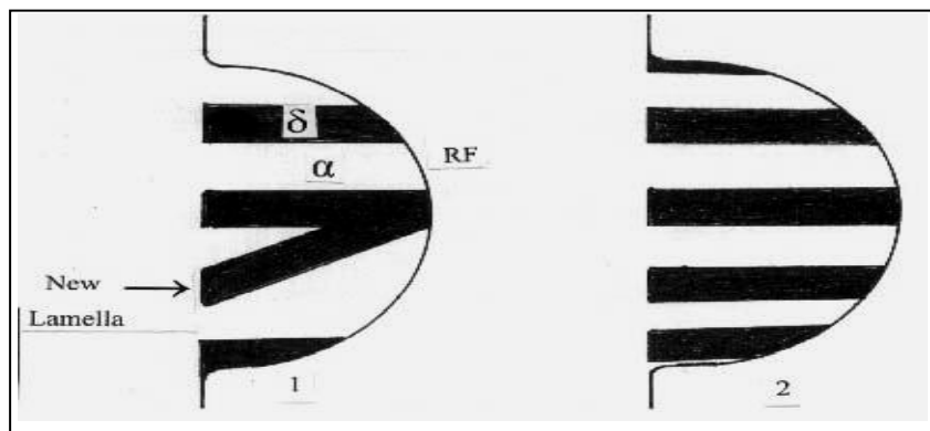
Figure 4. Illustration du mécanisme de branchement observé lors du vieillissement isotherme de l'alliage Cu-7,5 at. % In [41].
