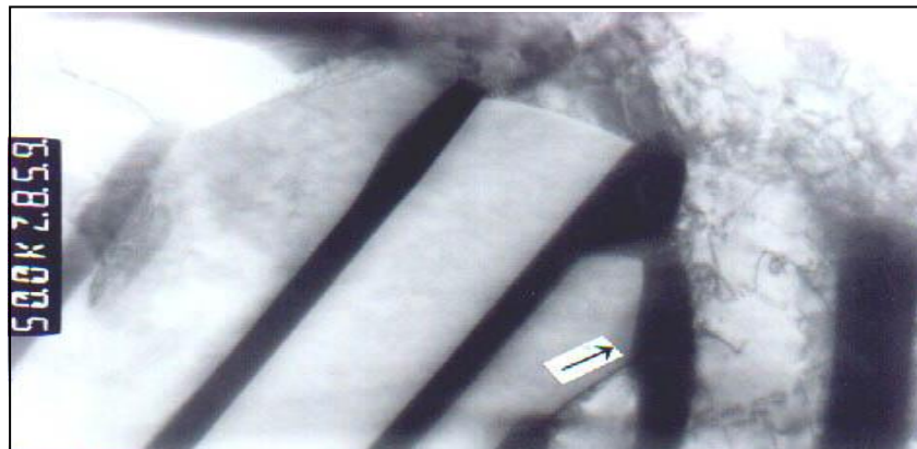
Figure 3. Mécanisme de branchement typique observé par MET lors du vieillissement isotherme de l'alliage Cu-7,5 at. % In à 400°C pendant 42 heures.
